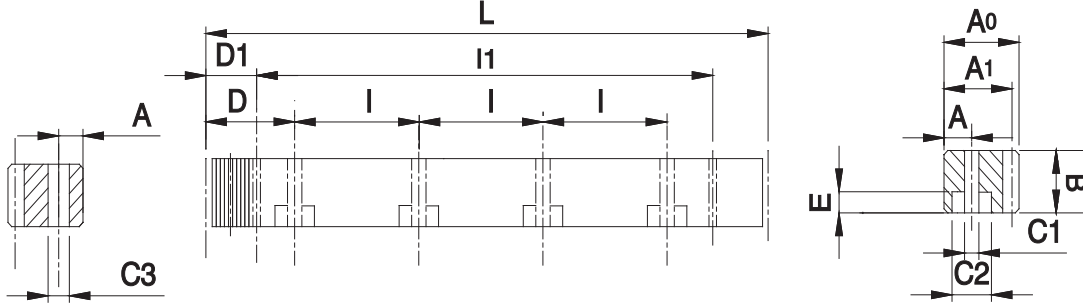
WINMAN DÜZ KREMAYERLER - WCSTMQ DIN 8e
