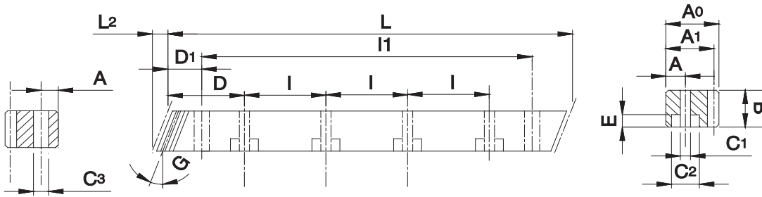
WINMAN HELİS KREMAYERLER (DELİKLİ) (SOFT)- WCHTMQ DIN 8e
